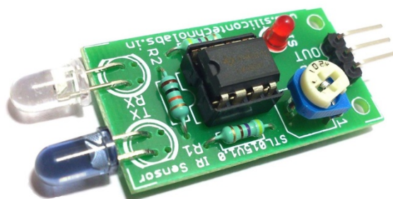
Fig 4.1.1 IR sensor
